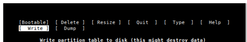
Abbildung 44: Partitionstabelle schreiben
