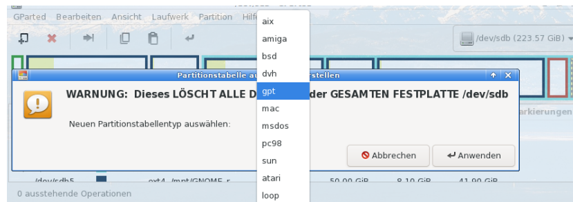
Abbildung 17: GParted Partitionstabelle
