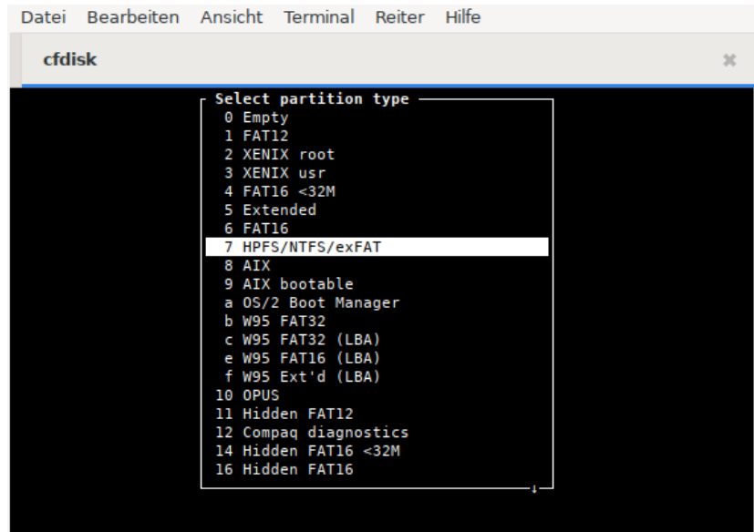
Abbildung 43: Partitionstyp auswählen
