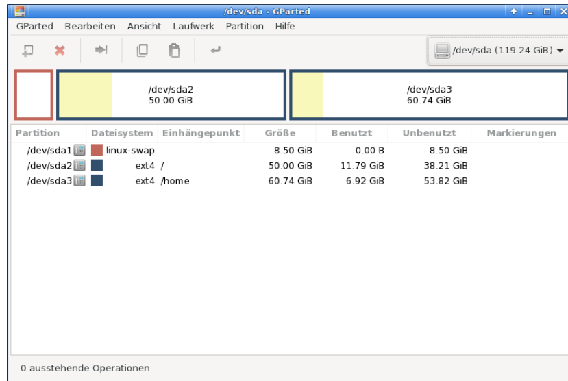
Abbildung 14: GParted Startfenster
