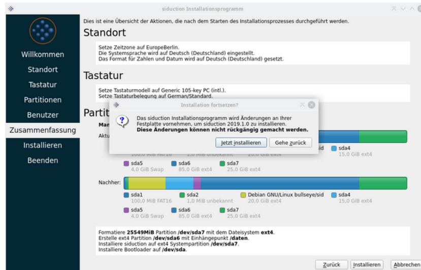
Abbildung 8: calamares Zusammenfassung
