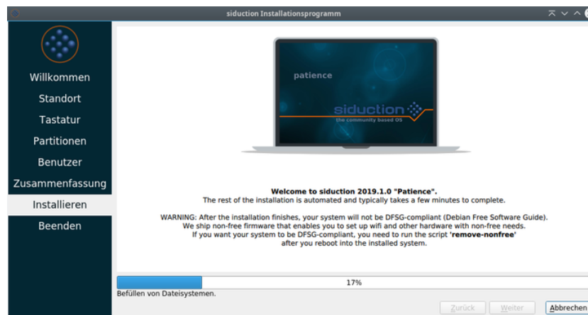
Abbildung 9: calamares Installieren
