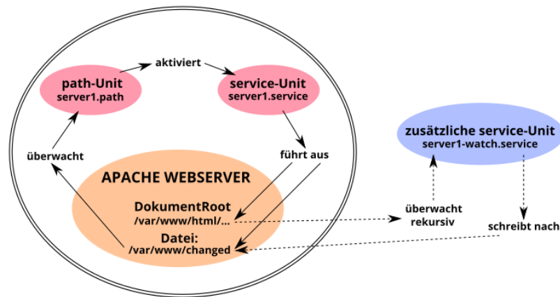
Abbildung 65: path-Unit Funktion
