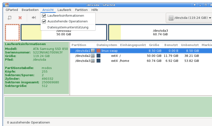
Abbildung 16: GParted Festplatteninformation
