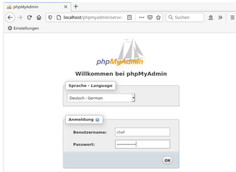
Abbildung 54: Loginfenster
