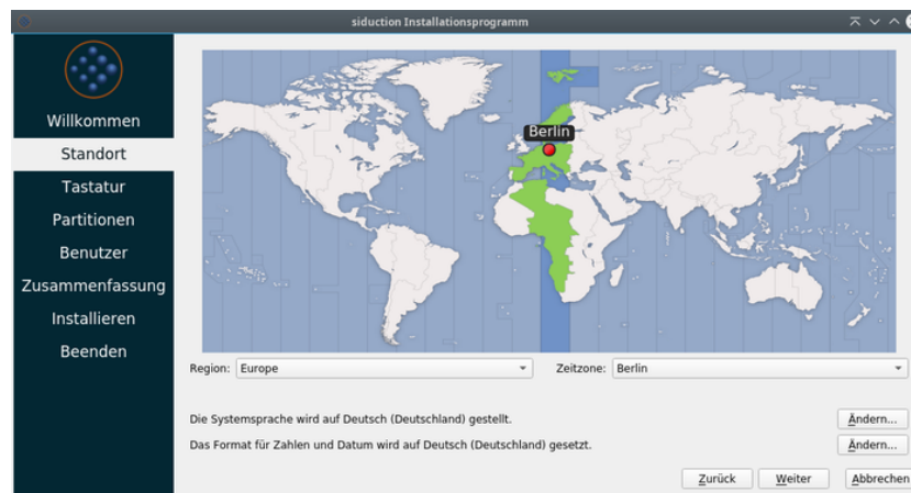
Abbildung 2: calamares Standort
