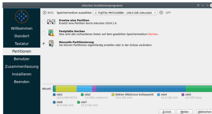
Abbildung 4: calamares Partitionen
