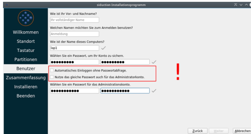
Abbildung 7: calamares Benutzer
