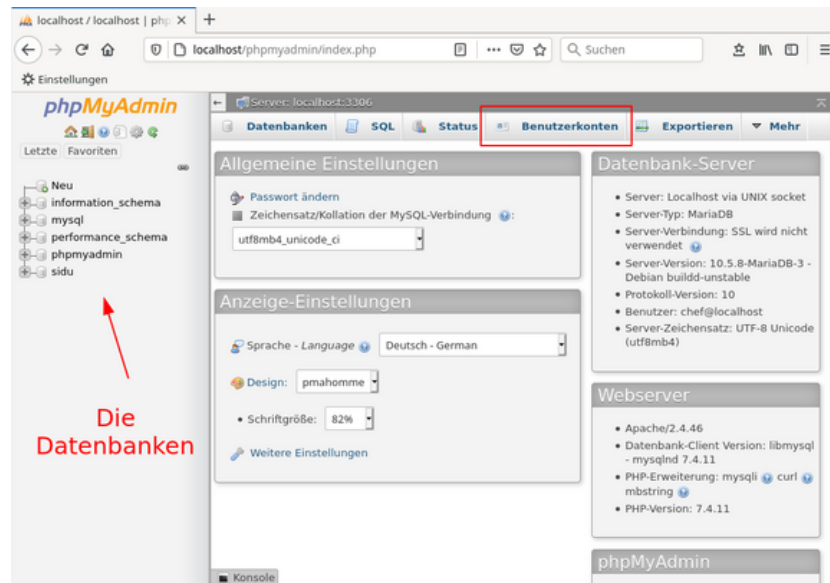
Abbildung 55: Startfenster
