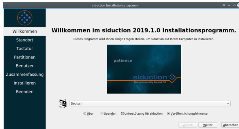
Abbildung 1: calamares Willkommen
