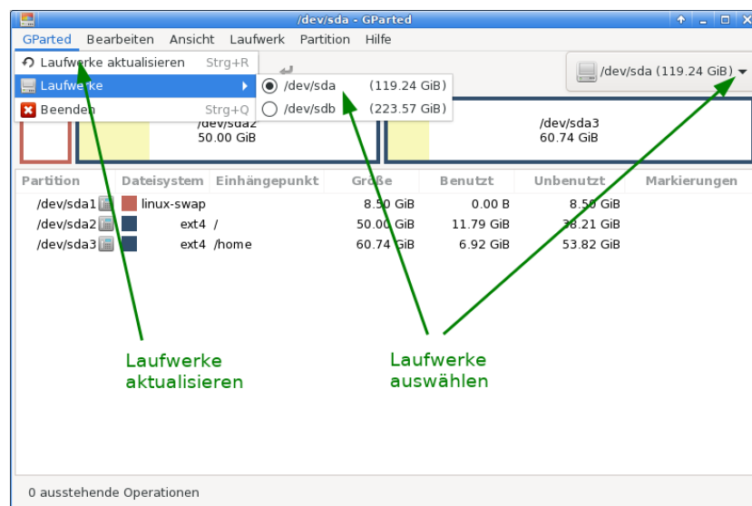
Abbildung 15: GParted Geräteübersicht
