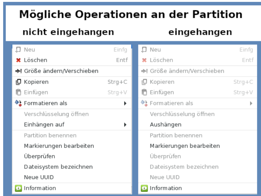
Abbildung 19: GParted Datenrettung
