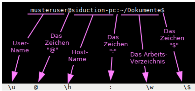
Abbildung 62: Prompt Code
