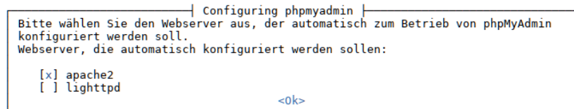
Abbildung 51: PHPMyAdmin Webserverauswahl
