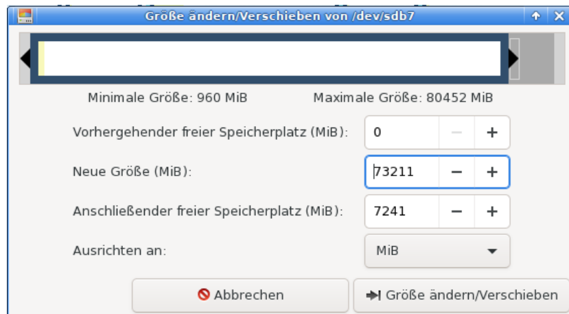
Abbildung 21: GParted Größenänderung
