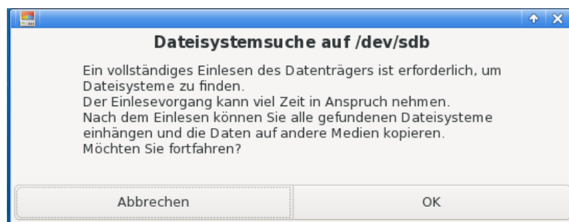
Abbildung 18: GParted Datenrettung
