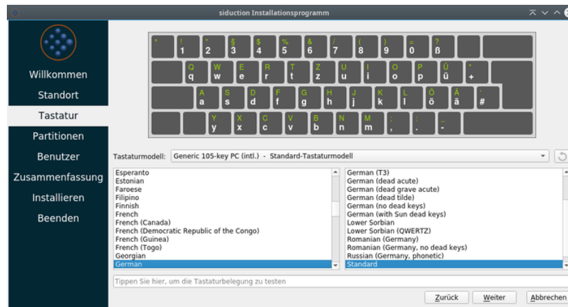
Abbildung 3: calamares Tastatur
