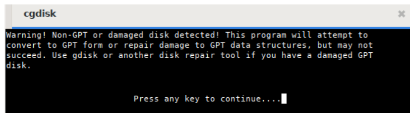
Abbildung 24: Warnmeldung
