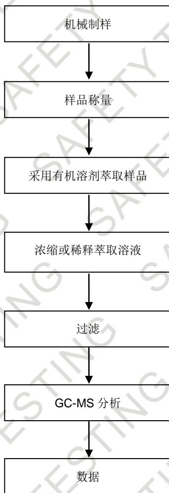
邻苯二甲酸酯 测试流程图
